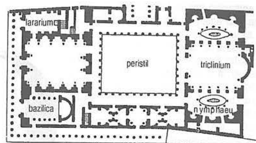
Planul Palatului Flaviiilor, sec. 1 d.H., Roma
