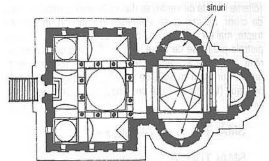
Biserica Mînăstirii Argeș, secțiune și plan
